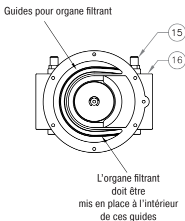
fig. a : Corps DN 15 ÷ DN 50 sans couvercle (4)
